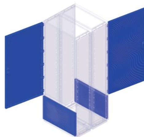
Armadio di profondità complessiva 660mm con 2 porte contrapposte 660mm overall depth enclosure with 2 opposing doors.
